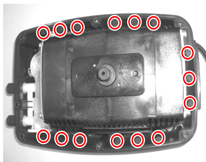
位置決めピンは15箇所あります。(○印部分)
